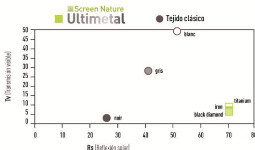
Resultados térmicos y ópticos del tejido Screen Nature Ultimetal comparados con los tejidos clásicos libre de PVC
